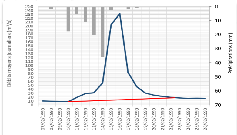
Figure C. Hydrogramme et hyétogramme de la crue de février 1990 de l'Orne à Rosselange et séparation des écoulements
