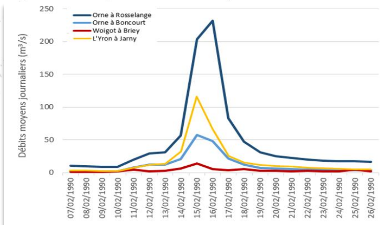
Figure B. Hydrogrammes de la crue de février 1990 sur l'Orne, l'Yron et le Woigot
