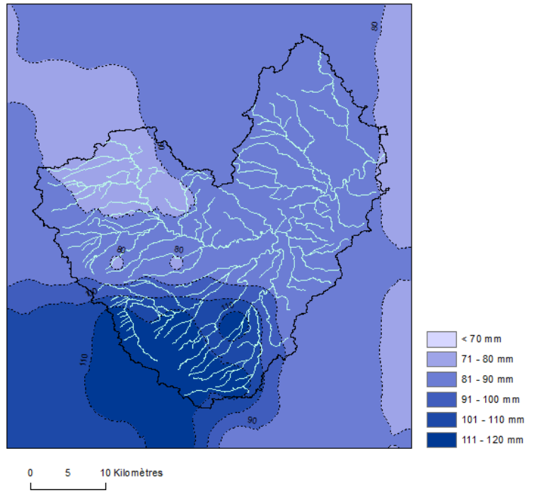
Figure D. Cumuls de précipitations sur le bassin versant de l'Orne du 10 au 14 février 1990
