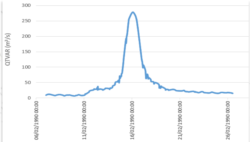
Figure A. Hydrogramme de la crue de février 1990 sur l'Orne à Rosselange (débits à pas de temps variables)
