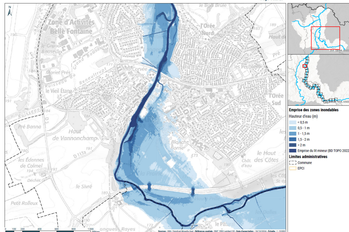
ATLAS DES ZONES INONDABLES PAR DÉBORDEMENT DE COURS D'EAU - CRUE D'OCCURRENCE TRENTENNALE (Q30) Bassin versant de la Seille
