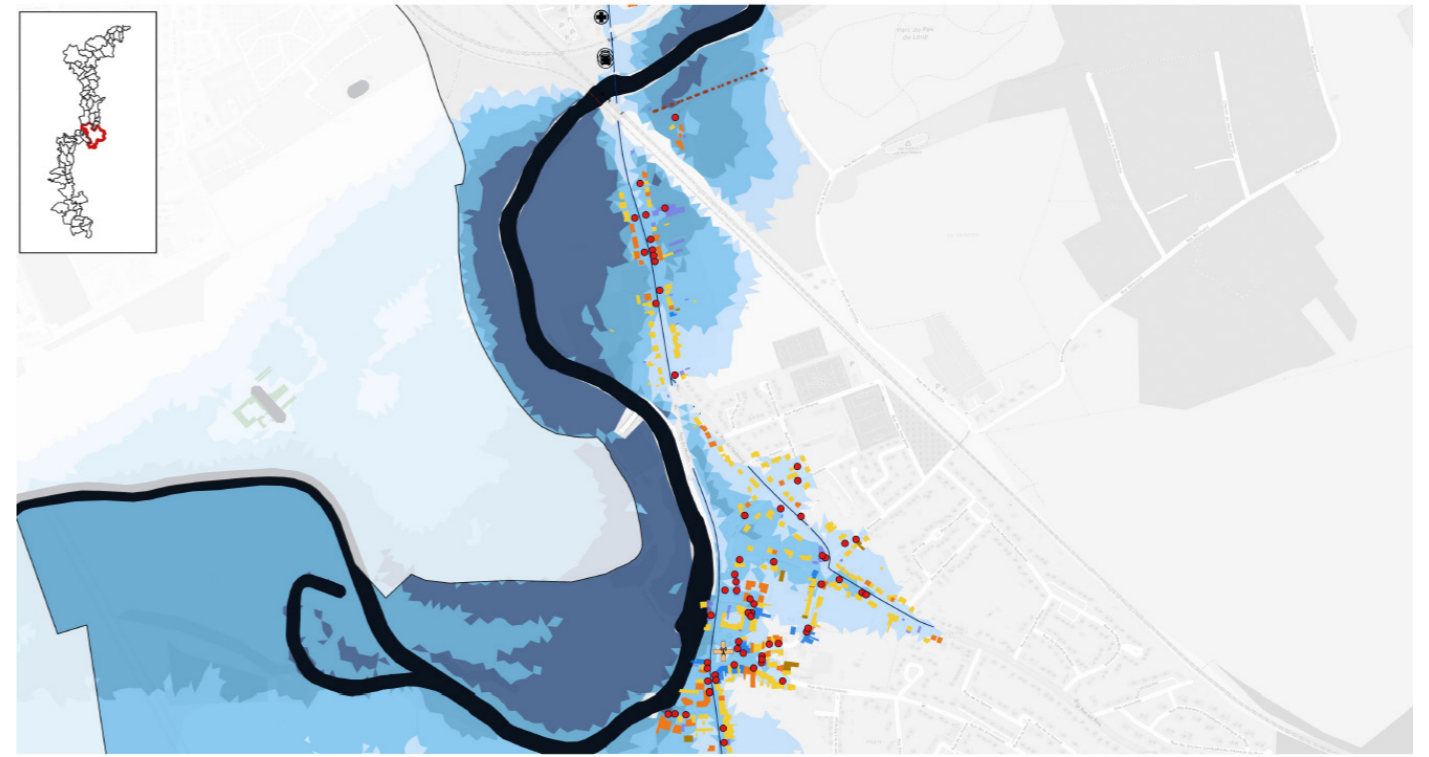
Carte du risque Q1000 - METZ
